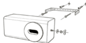
▲ Montage mit Haltebügel
