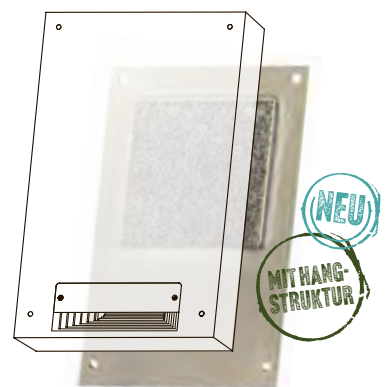
▲ 2WI mit optionaler Rückwand (Bestell-Nr. 00 778/0)
