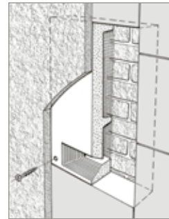
▲ Einbaubeispiel, rückseitig offen ohne Rückwand
