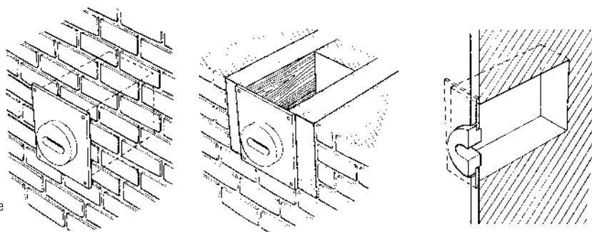
Montagebeispiele
