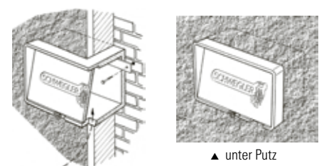
▲ eingebaut in die Isolierung mit Halteleistenbefestigung
