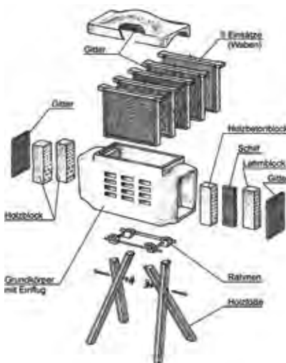
▲ Einzelteile (Übersicht)
